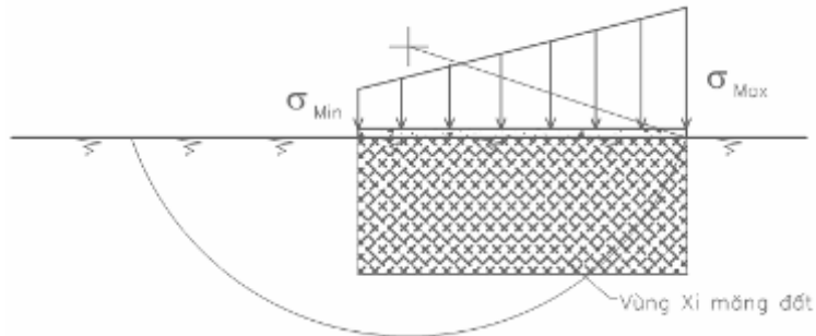
Hình D.1 - Sơ đồ tính toán theo phương pháp mặt trượt trụ tròn
