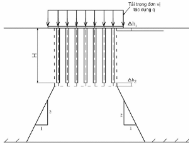
Hình E.7 - Sơ đồ tính toán biến dạng
