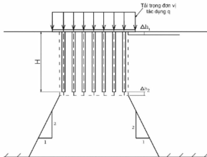
Hình D.3 - Sơ đồ tính toán biến dạng
